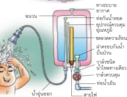
ส่วนประกอบของเครื่องทำน้ำอุ่นที่มีความจุน้อย
